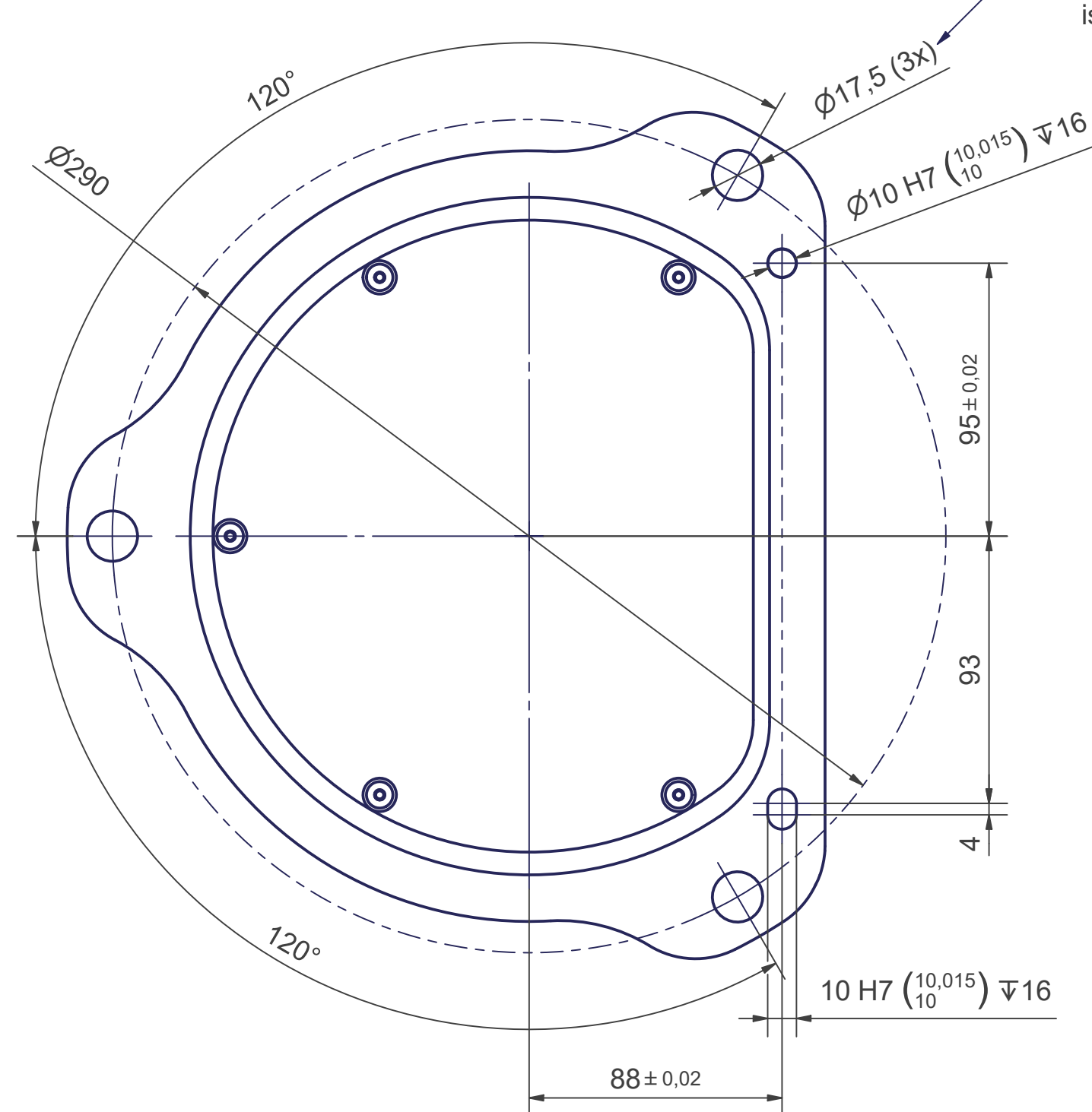
C (1 : 2) Base frame
